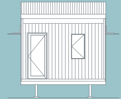
4 ELEVATION 1B ENSUITE
