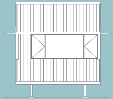
3 ELEVATION 1B ENSUITE
